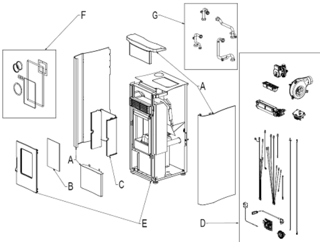
Fig. 1 - Geëxplodeerde tekening
